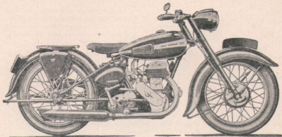
Moto HCTL (côté distribution)
